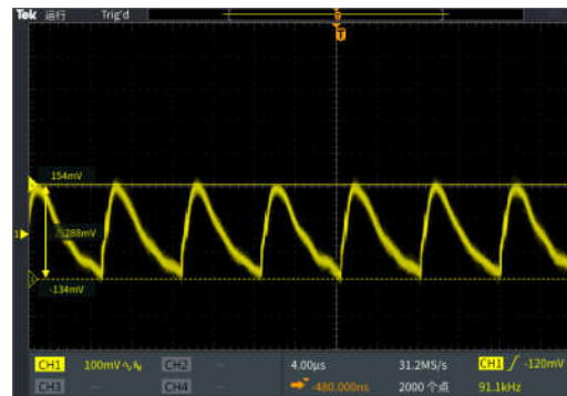
图五推荐测试方法为 \Delta V_{pp}=288\text{mV}
